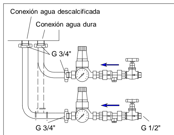
Kit de conexión completo 2 x código 172449 incluye: 2 válvula de retención 2 válvula reductora de presión 2 Llave de paso
