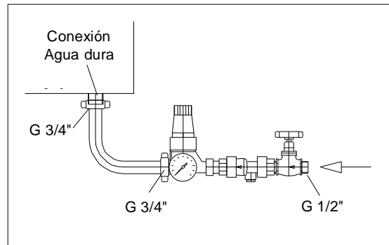
Kit de conexión completo código 172449 incluye: 1 válvula de retención 1 válvula reductora de presión 1 Llave de paso
