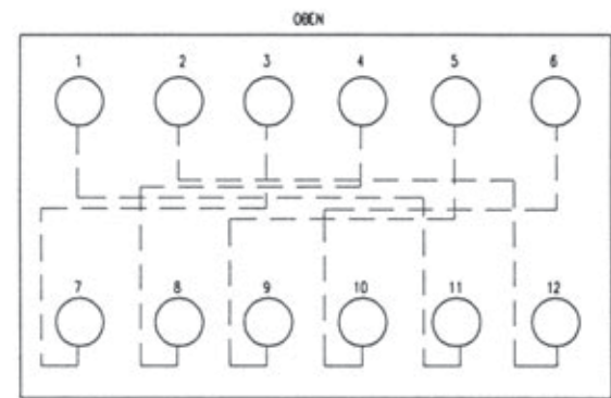
Conexionado resistencias (E2) 230 V
