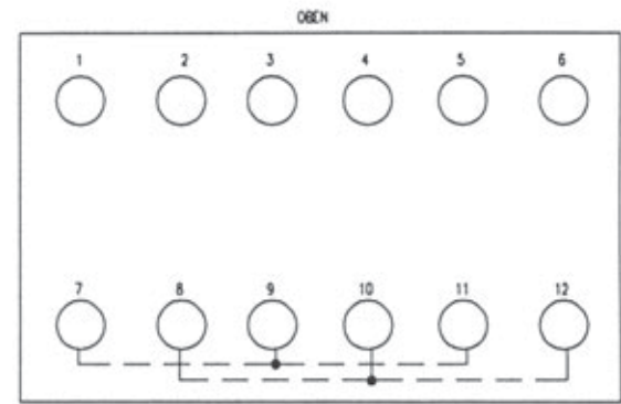
Conexionado resistencias (E2) 400 V
