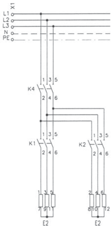
400V 3PN AC 15 kW (6*2.5kW)
