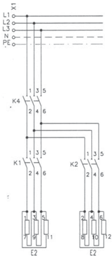
230V 3P AC 15 kW (6*2.5kW)
