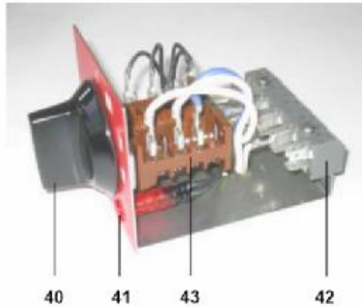
Steuerung mit Timer Commande avec minuterie Timer control
